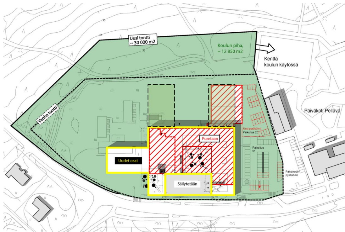
Kuva 10 VE2 tontinkäyttösuunnitelma
