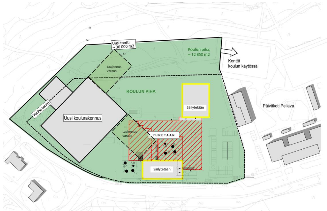
Kuva 16 VE3B Tontinkäyttösuunnitelma
